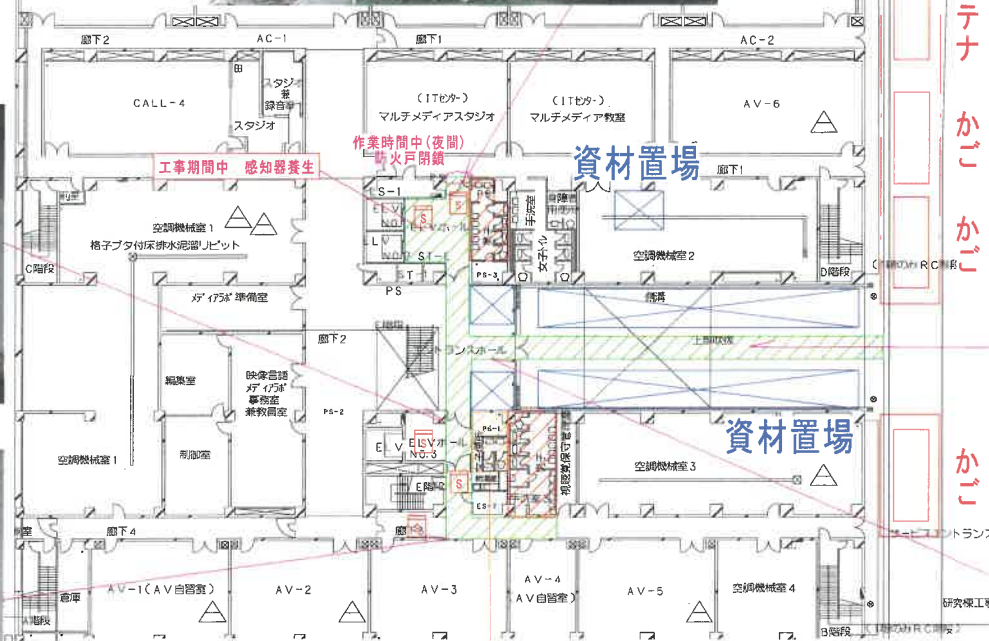
外部養生図
