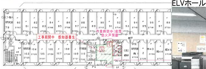
6階平面図
